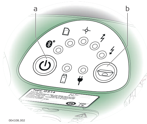
a) ON/OFF button b) Function button
